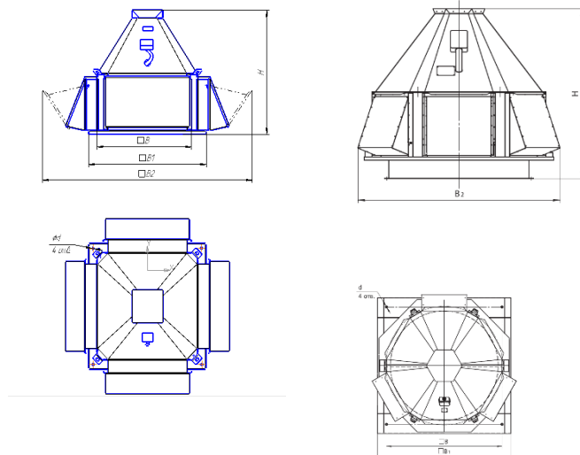
Рисунок 1 – Загальний вигляд вентиляторів типу UKROS–DU (DUV)
