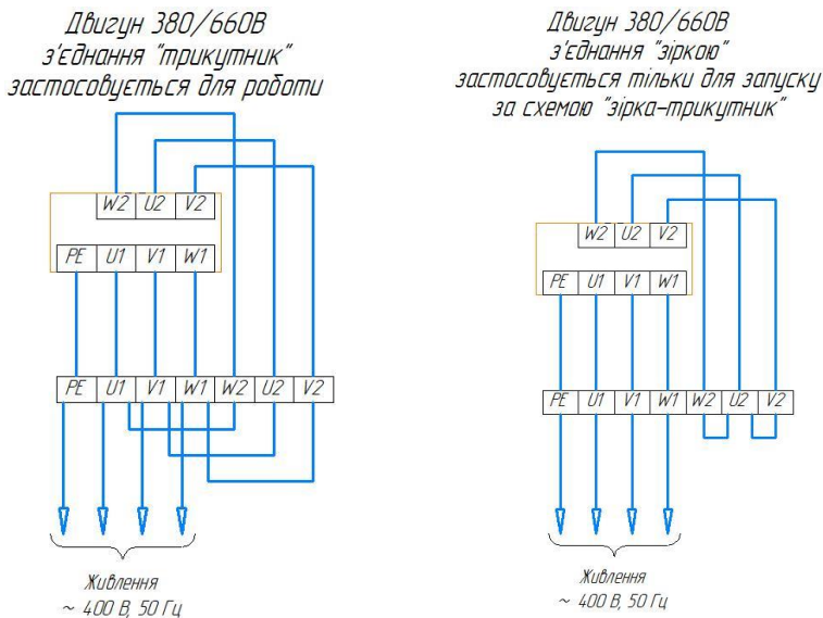
Рисунок 2. Схеми підключення двигуна
