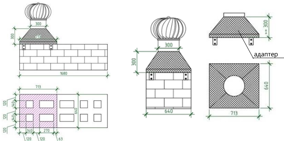
Рисунок 4 Приклад монтажу дефлектора на вентиляційному каналі
