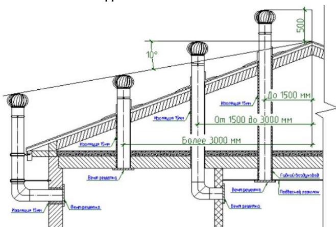
Рисунок 5 Пример монтажа дефлектора на скатных дахах
