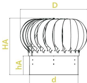
Рисунок 2 Загальний вид дефлектору типу AVD з муфтовим та ніпельним з'єднанням
