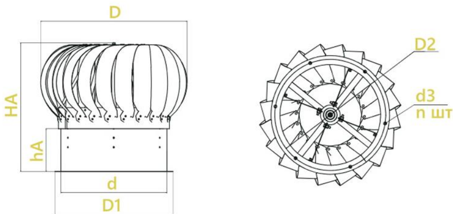
Рисунок 1 Загальний вид дефлектору типу AVD з фланцевим з'єднанням
